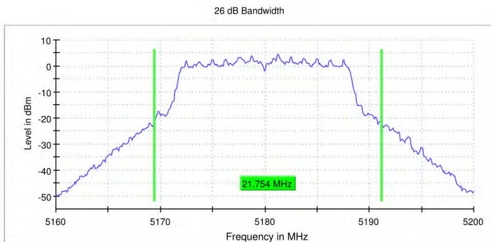
11A_Ant0_5180
