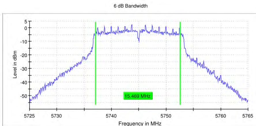
11A_Ant0_5745
