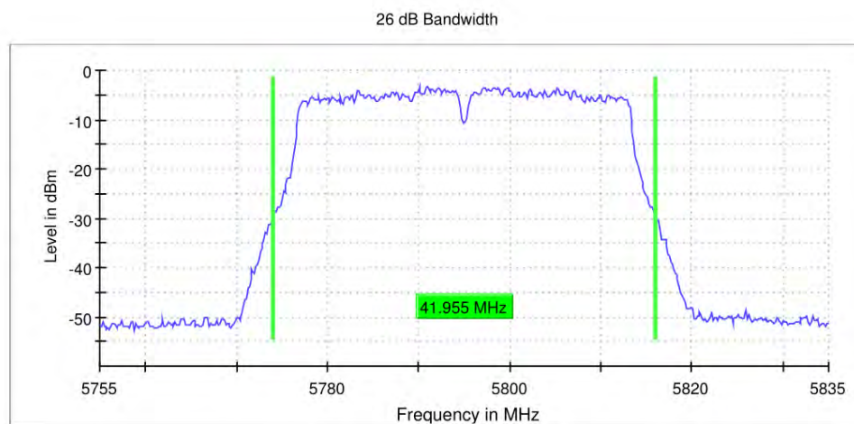
11N40_Ant0_5795
