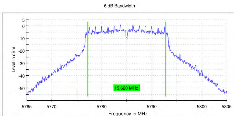
11A_Ant0_5785
