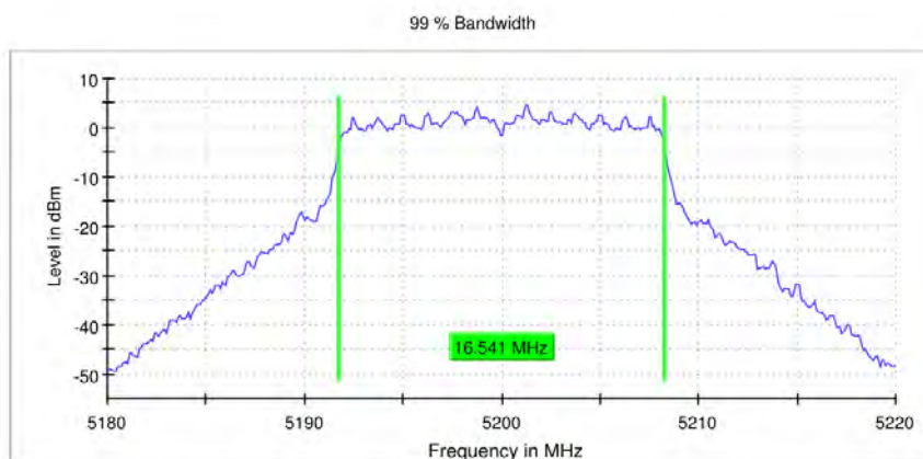
11A_Ant0_5200
