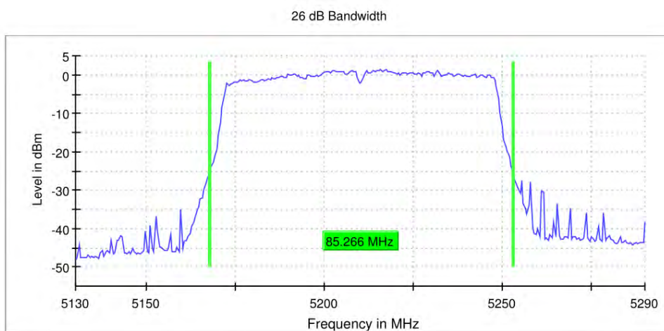
11AC80_Ant0_5210
