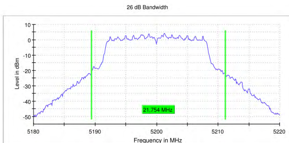
11A_Ant0_5200
