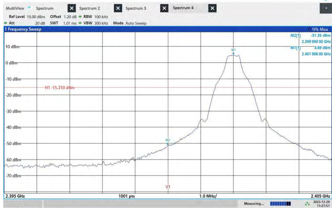
DH5_Ant1_Low_2402
