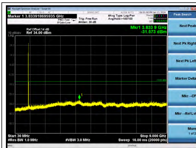
CDMA BC0-1013-5-30~9000MHz-PASS
