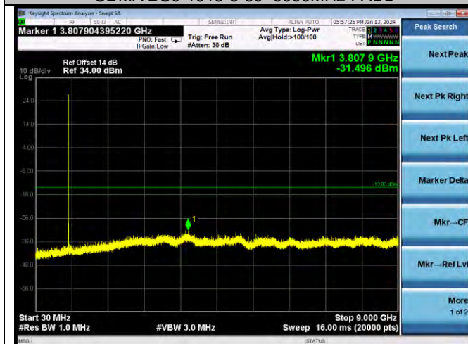
CDMA BC0-384-5-30~9000MHz-PASS
