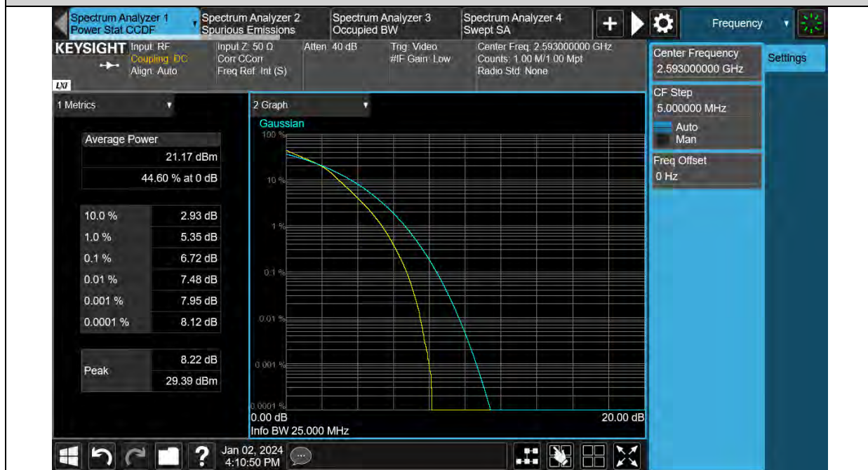
Band41-20MHz-16QAM-41490-1RB#0
