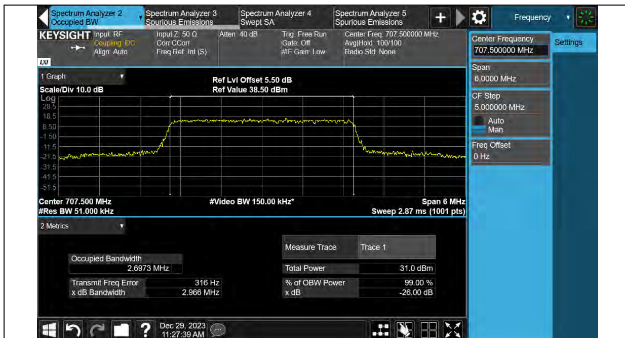
Band12-3MHz-QPSK-23165-15RB#0
