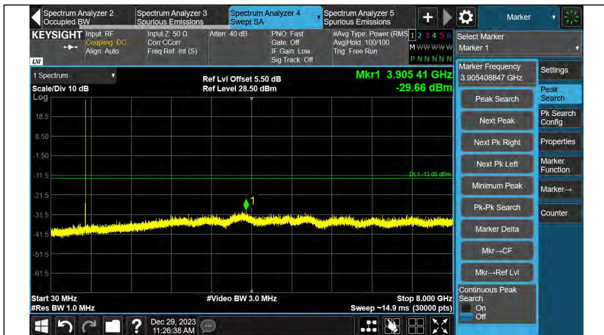
Band12-3MHz-QPSK-23025-1RB#0-30~8000MHz
