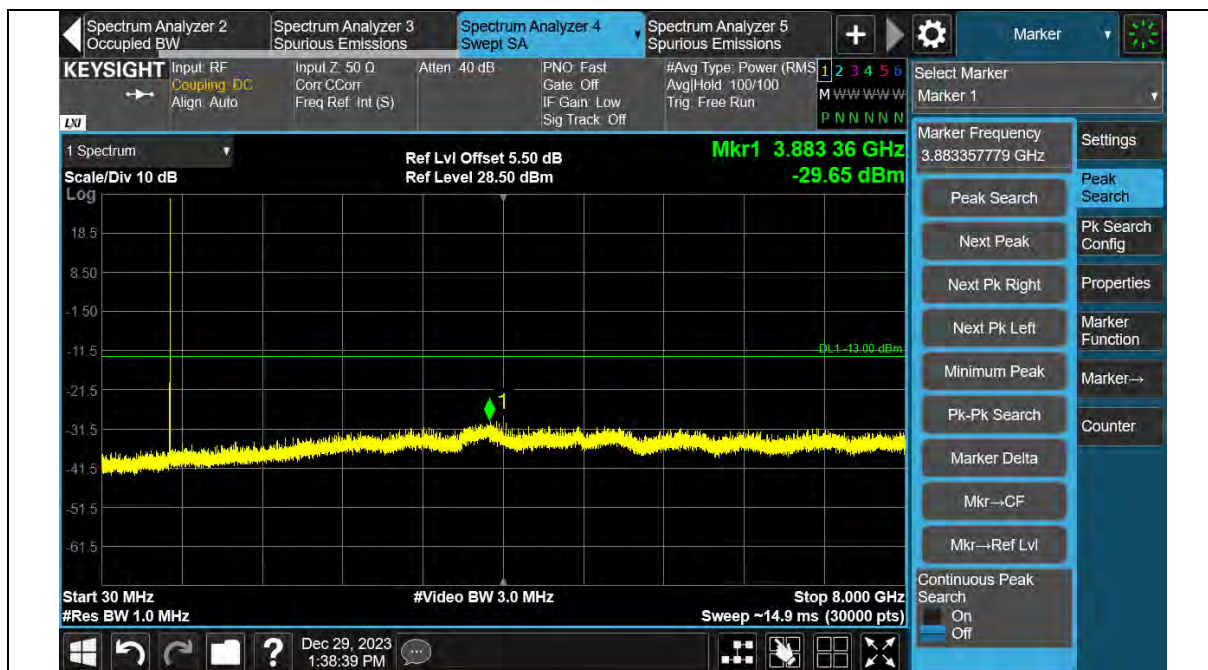
Band12-3MHz-QPSK-23165-1RB#0-30~8000MHz
