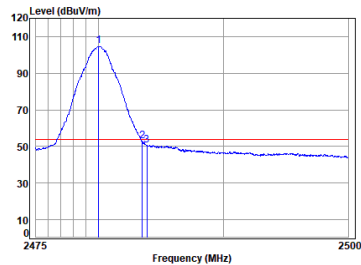
PIFA ANT BLE_2M_TX_CH_39_Vertical-Avg
