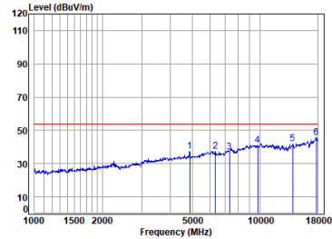
PIFA ANT BLE_2M_TX_CH_19_Horizontal-Avg
