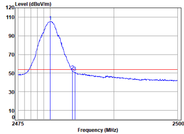
PIFA ANT BLE_2M_TX_CH_39_Horizontal-Avg
