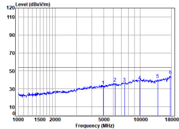
FPC ANT BLE_2M_TX_CH_39_Vertical-Avg
