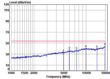
FPC ANT BLE_2M_TX_CH_39_Horizontal-Avg
