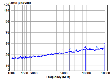
FPC ANT BLE_2M_TX_CH_19_Vertical-Avg
