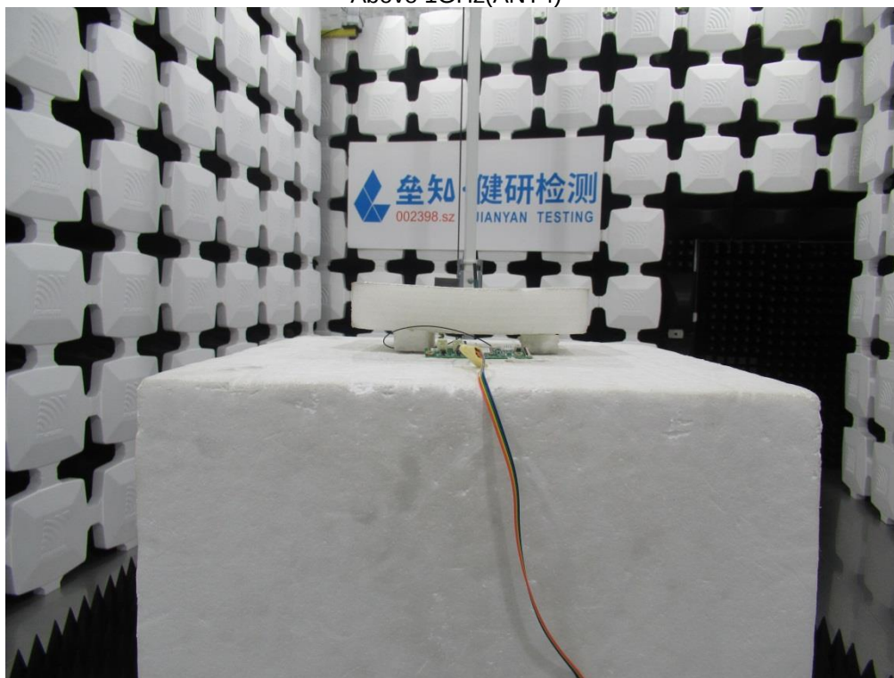
Above 1GHz(ANT4)
