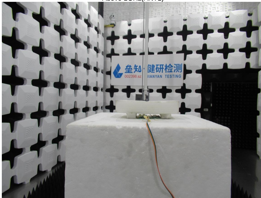
Above 1GHz(ANT1)
