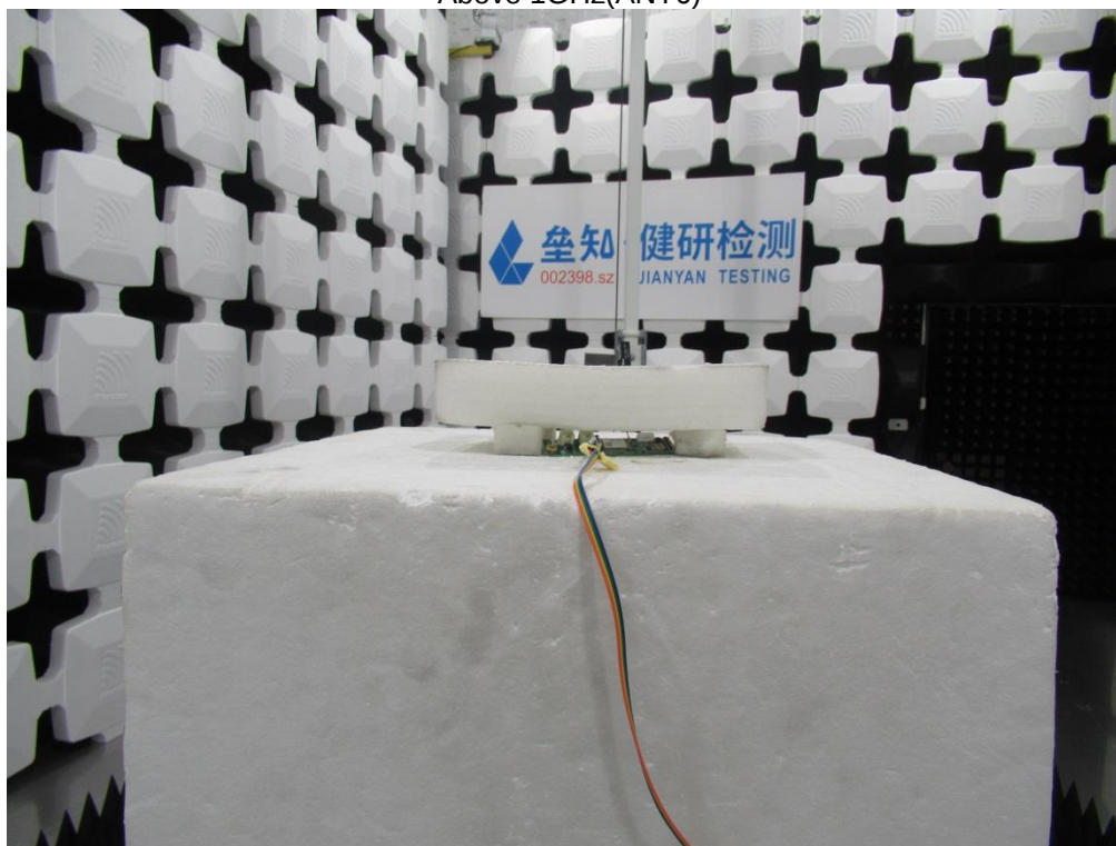
Above 1GHz(ANT6)
