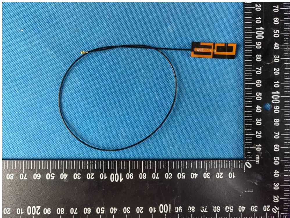
Optional Antenna 3 RD542109NB86-3
