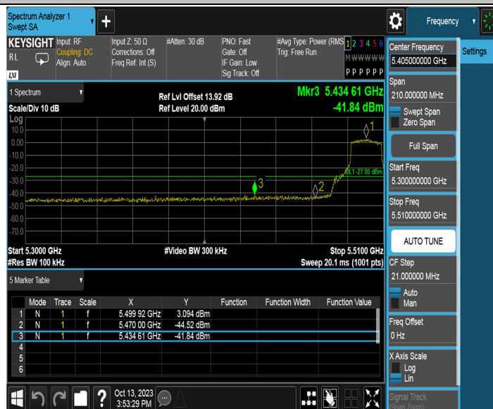
11AC20MIMO_Ant2_Low_5500
