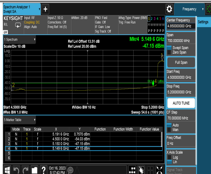
11AC40MIMO_Ant1_Low_5190_AV
