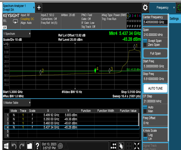
11AC20MIMO_Ant2_Low_5500_Peak
