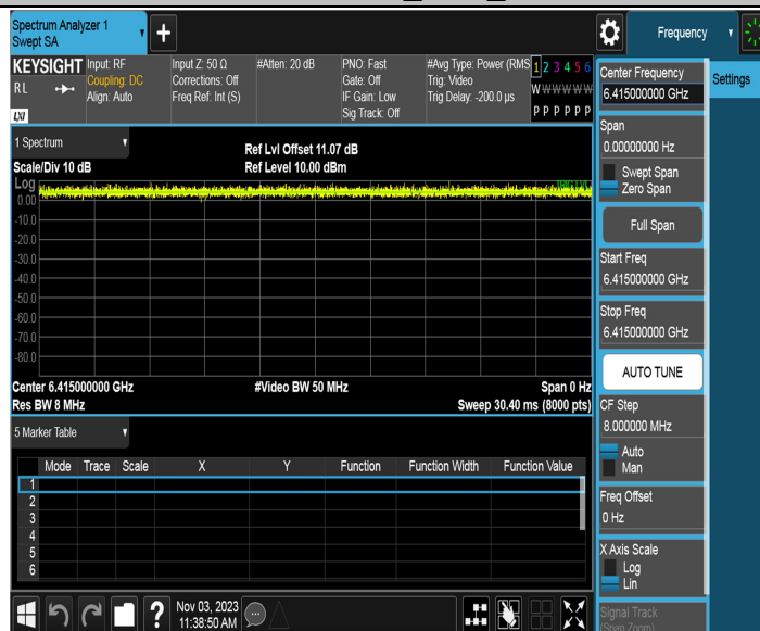
11AX20MIMO_Ant1_6415
