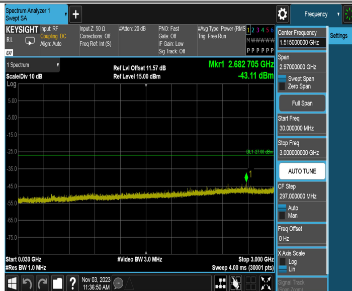
11AX20MIMO_Ant2_6175_30~3000
