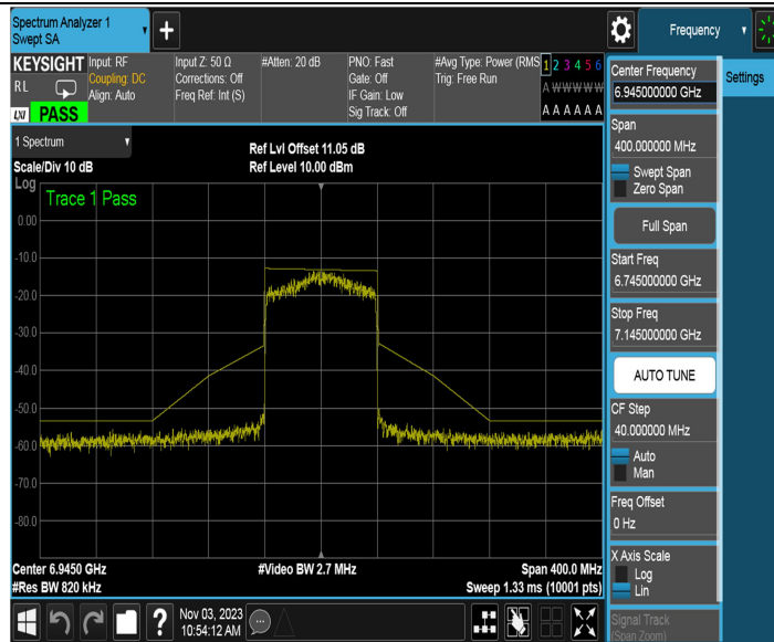
11AX80MIMO_Ant2_6945
