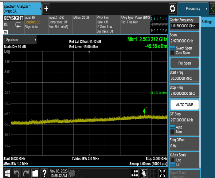
11AX80MIMO_Ant2_6945_30~3000
