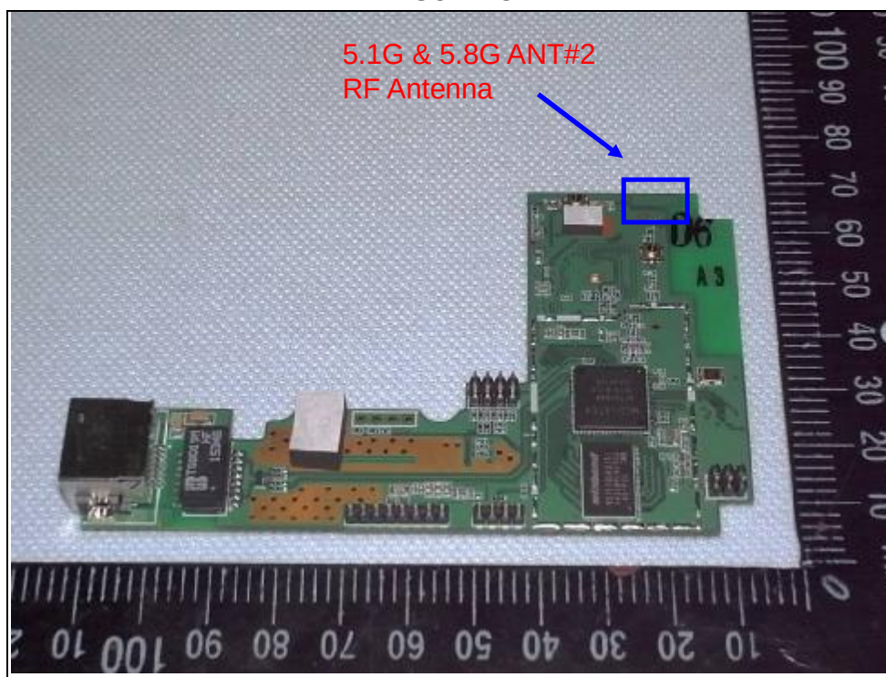
MLWG3 : PCB-2
