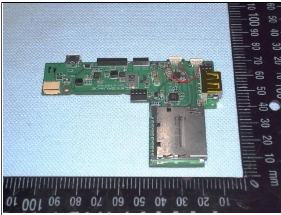
MLWG3/64 : PCB-1
