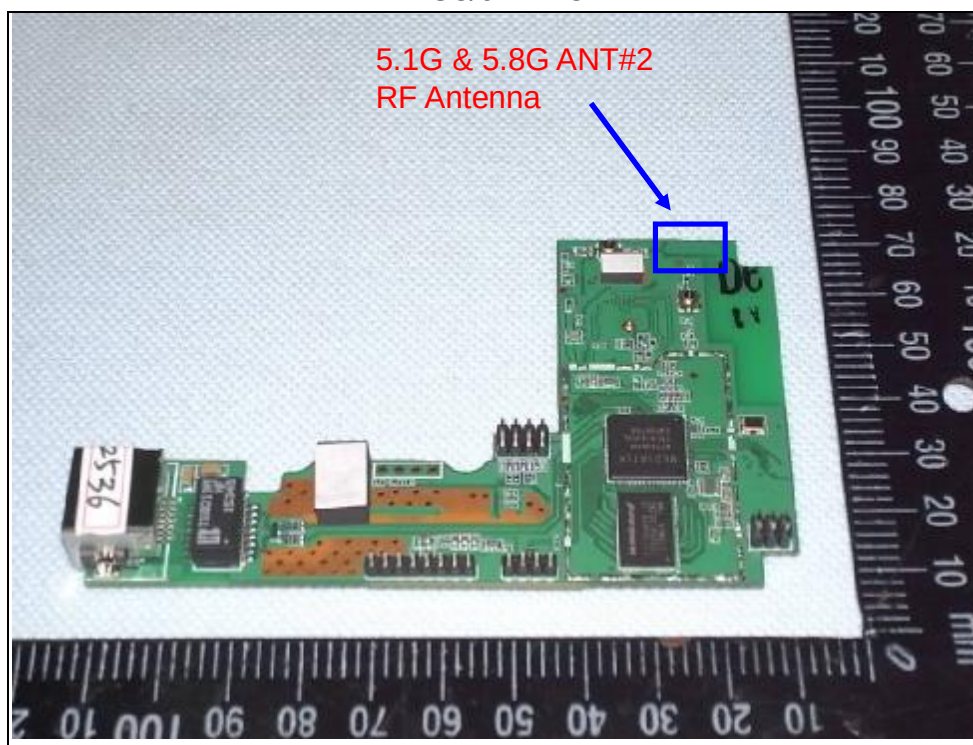
MLWG3/64 : PCB-2
