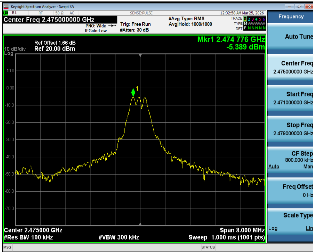
Band Edge NVNT 2.4G 2475MHz Ant1 Ref
