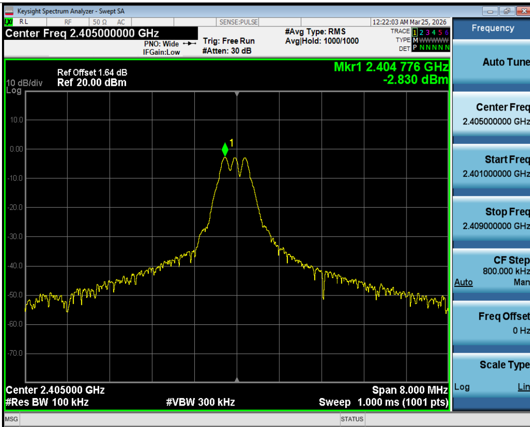
Band Edge NVNT 2.4G 2405MHz Ant1 Ref
