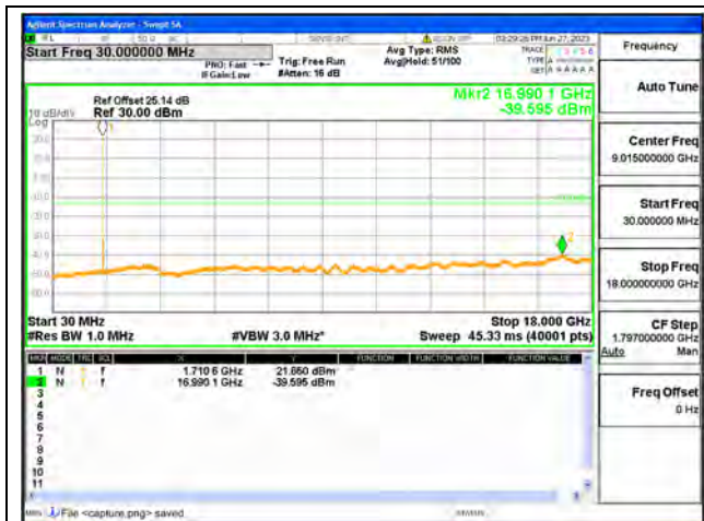
Band4 / 5MHz / Low CH / QPSK
