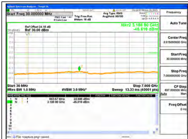
Band71 / 5MHz / Low CH / QPSK
