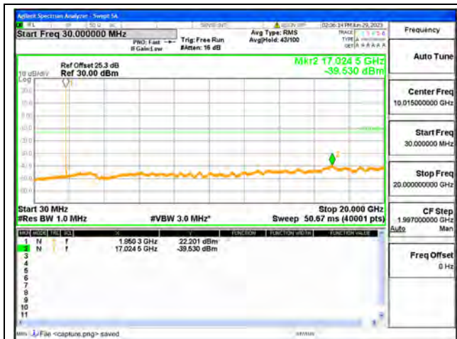
Band25 / 5MHz / Low CH / QPSK
