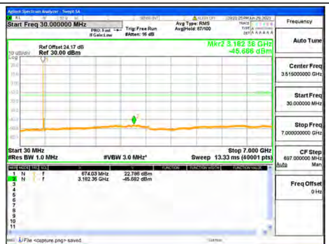
Band71 / 15MHz / Mid CH / QPSK
