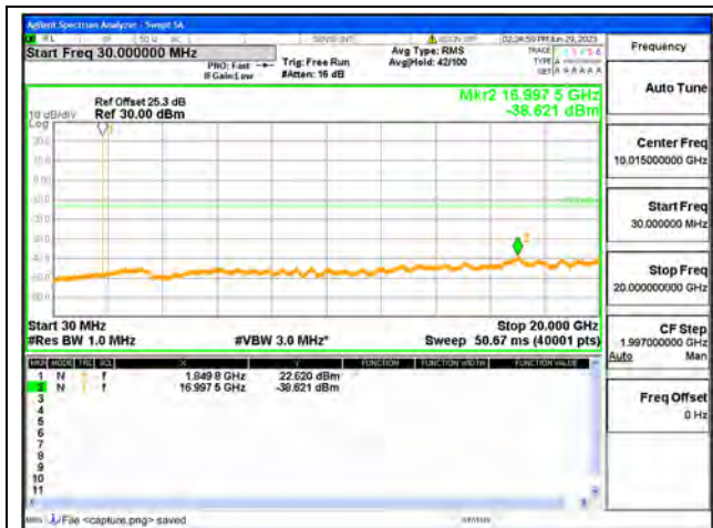
Band25 / 1.4MHz / Low CH / QPSK
