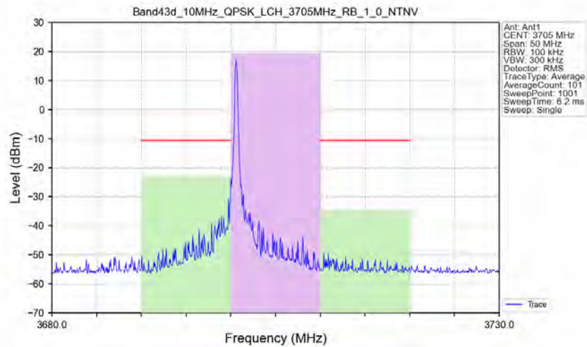
Band43d_10MHz_QPSK_LCH_3705MHz_RB_1_0_NTNV
