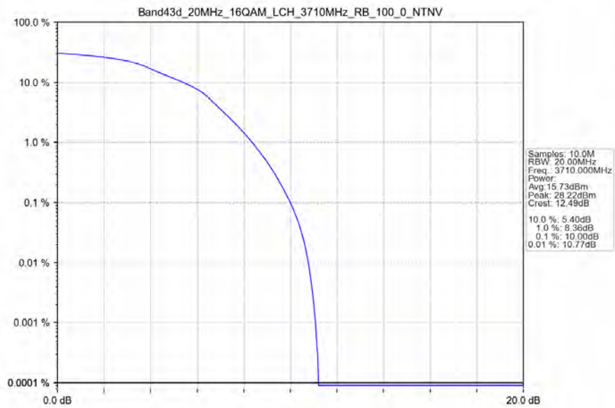
Band43d_20MHz_16QAM_LCH_3710MHz_RB_100_0_NTNV
