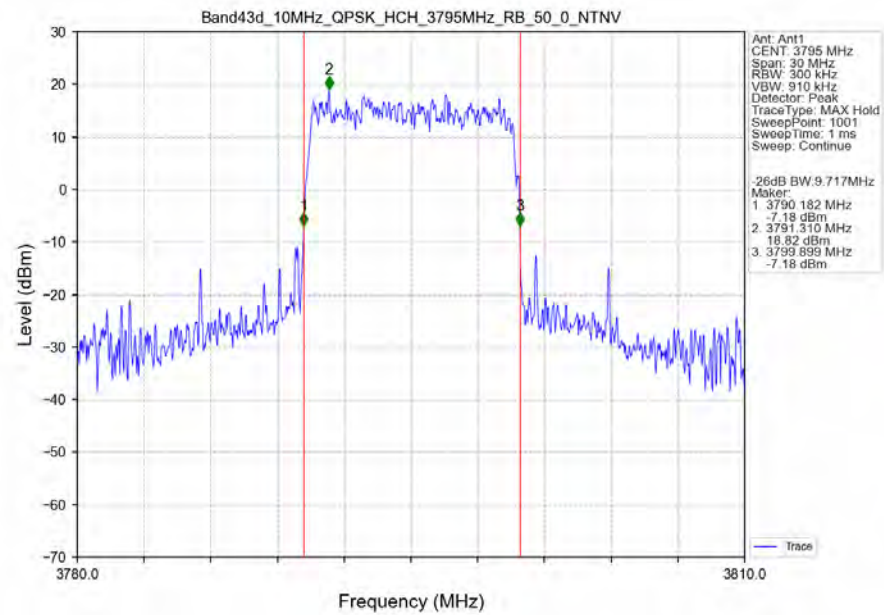
Band43d_10MHz_QPSK_HCH_3795MHz_RB_50_0_NTNV
