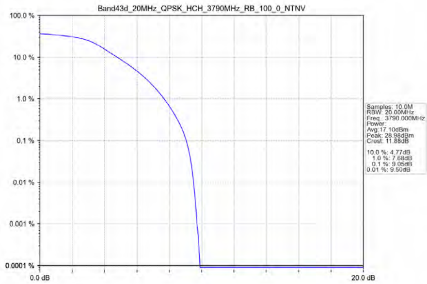
Band43d_20MHz_QPSK_HCH_3790MHz_RB_100_0_NTNV
