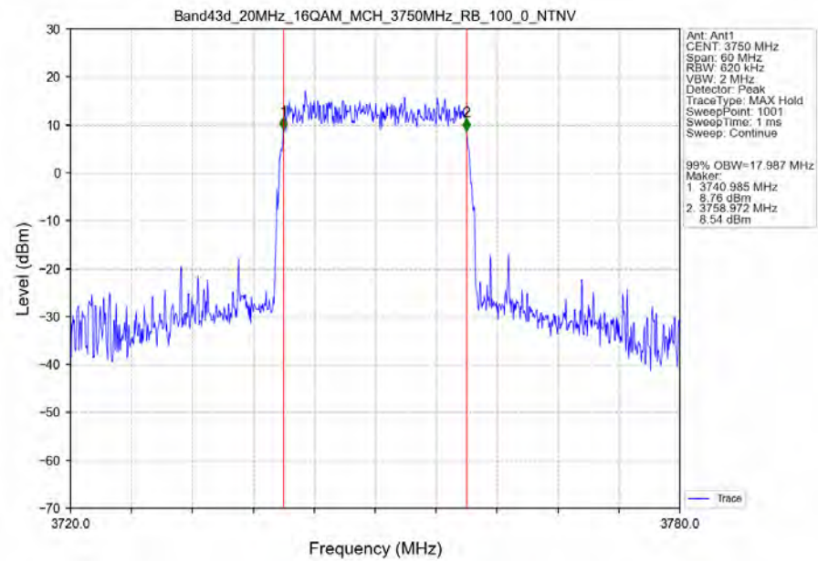
Band43d_20MHz_16QAM_MCH_3750MHz_RB_100_0_NTNV
