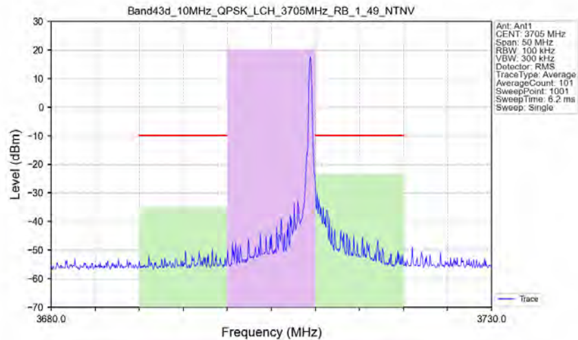
Band43d_10MHz_QPSK_LCH_3705MHz_RB_1_49_NTNV
