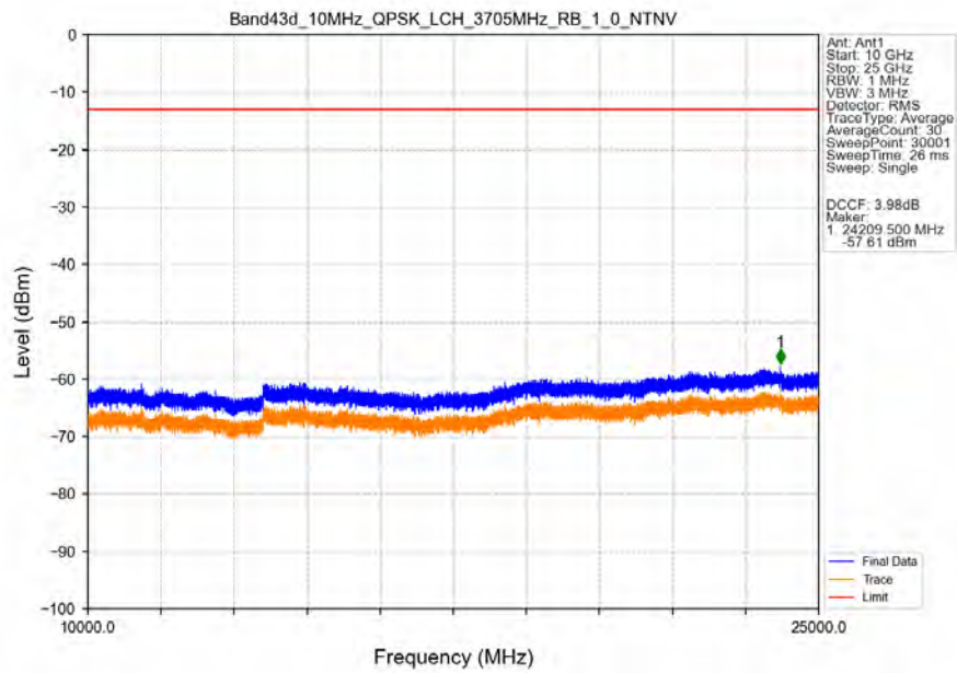
Band43d_10MHz_QPSK_LCH_3705MHz_RB_1_0_NTNV
