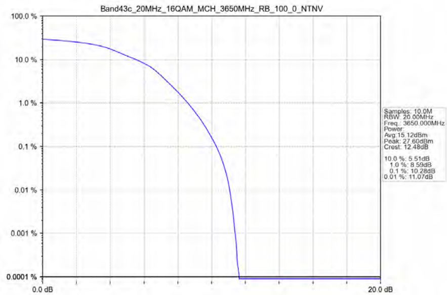
Band43c_20MHz_16QAM_MCH_3650MHz_RB_100_0_NTNV
