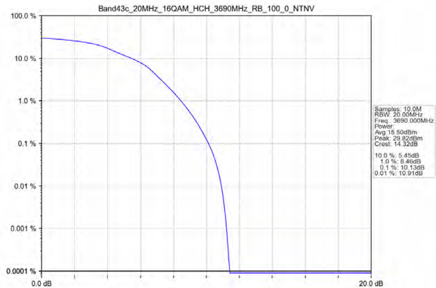
Band43c_20MHz_16QAM_HCH_3690MHz_RB_100_0_NTNV
