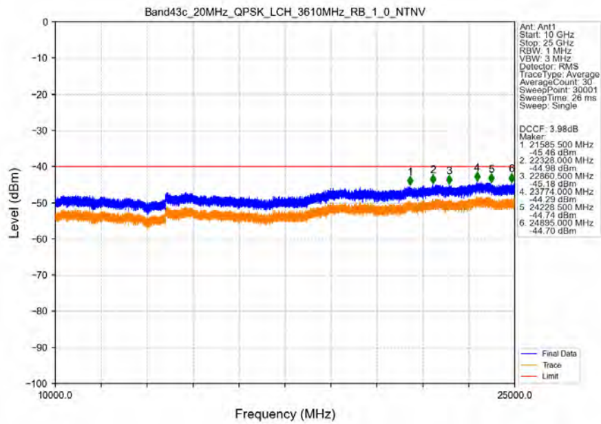
Band43c_20MHz_QPSK_LCH_3610MHz_RB_1_0_NTNV
