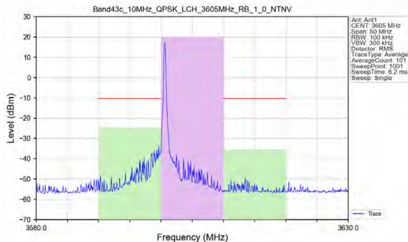
Band43c_10MHz_QPSK_LCH_3605MHz_RB_1_0_NTNV
