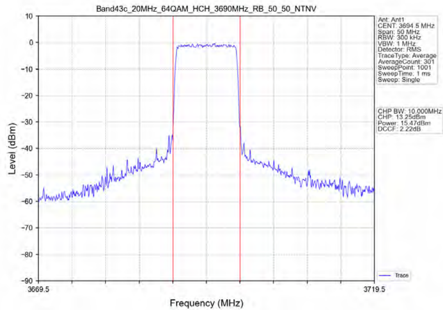
Band43c_20MHz_64QAM_HCH_3690MHz_RB_50_50_NTNV
