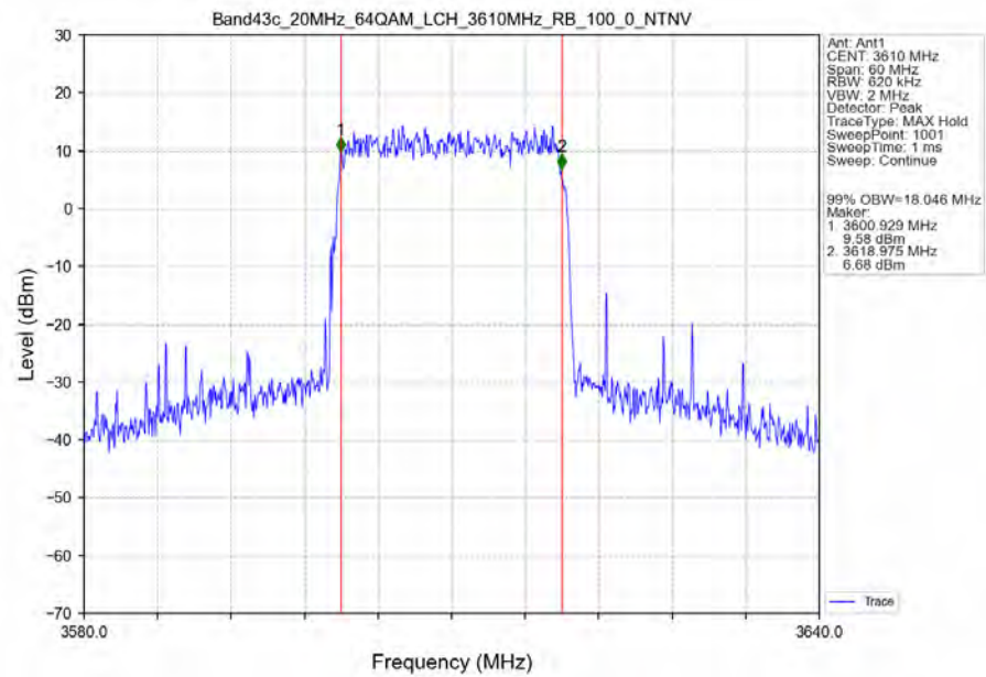
Band43c_20MHz_64QAM_LCH_3610MHz_RB_100_0_NTNV
