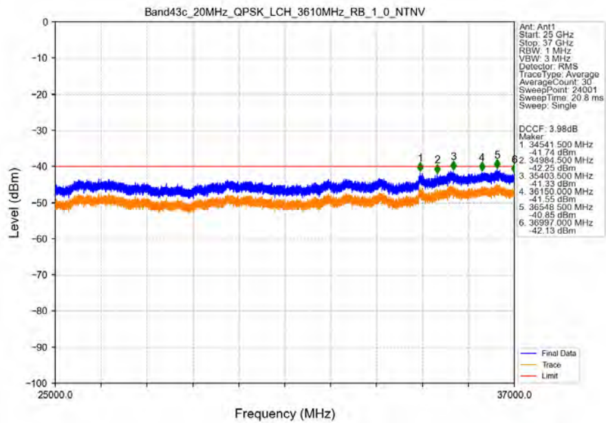
Band43c_20MHz_QPSK_LCH_3610MHz_RB_1_0_NTNV
