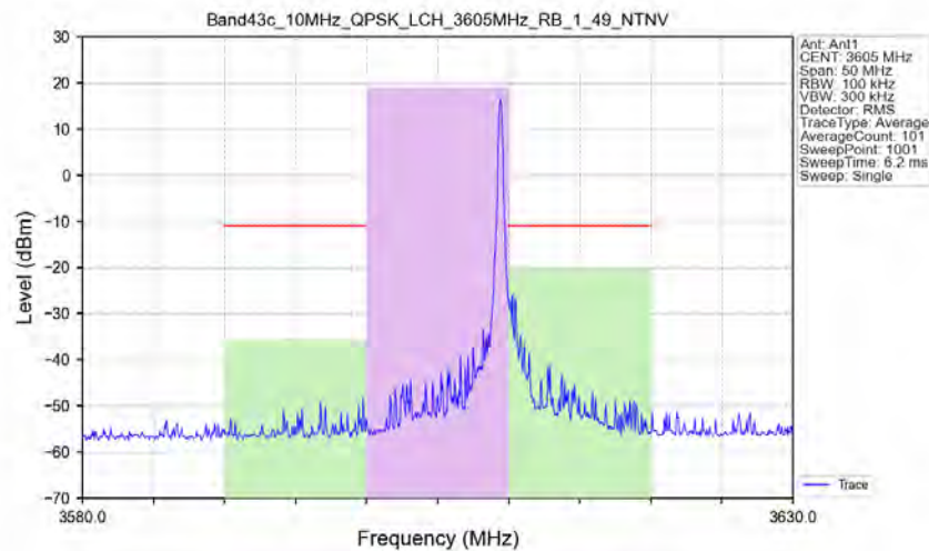
Band43c_10MHz_QPSK_LCH_3605MHz_RB_1_49_NTNV
