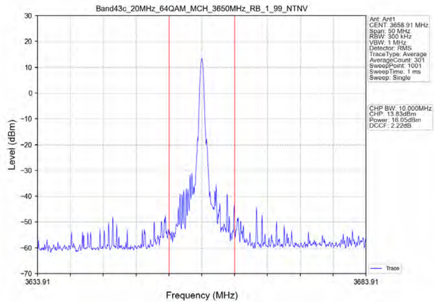
Band43c_20MHz_64QAM_MCH_3650MHz_RB_1_99_NTNV
