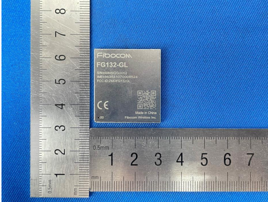
FG132-GL(LGA)
