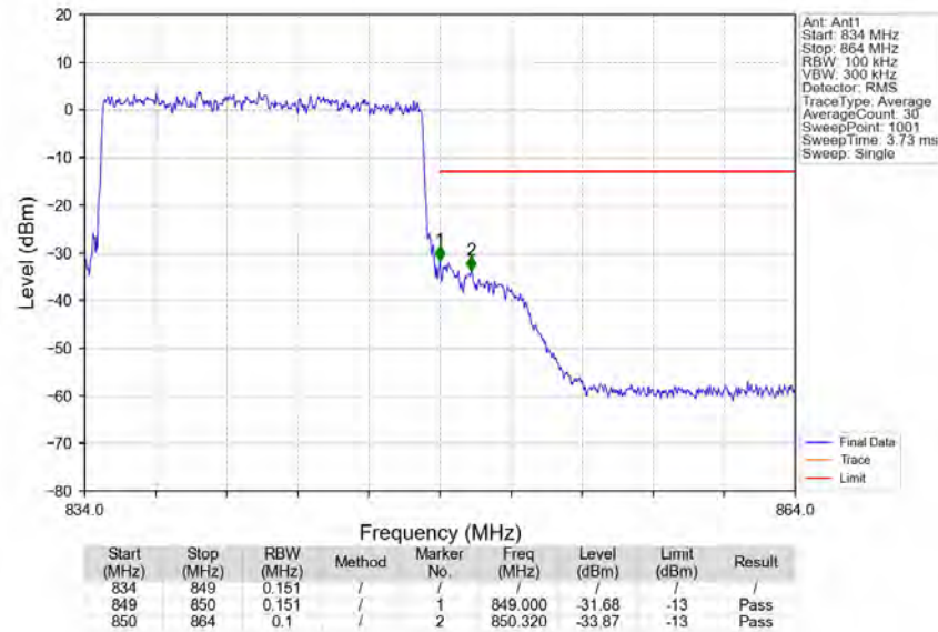
Band26c_15MHz_QPSK_HCH_841.5MHz_RB_75_0_NTNV
