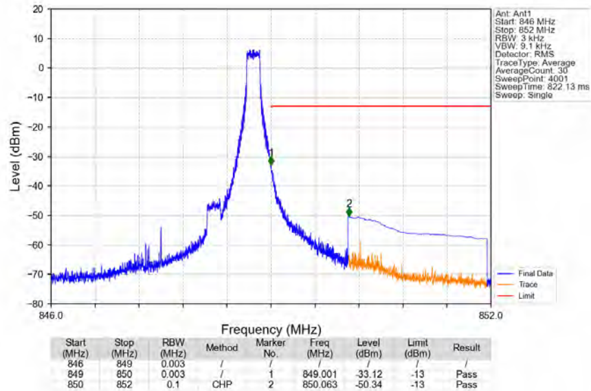
Band26b 3MHz 16QAM HCH 847.5MHz_RB_1_14_NTNV
