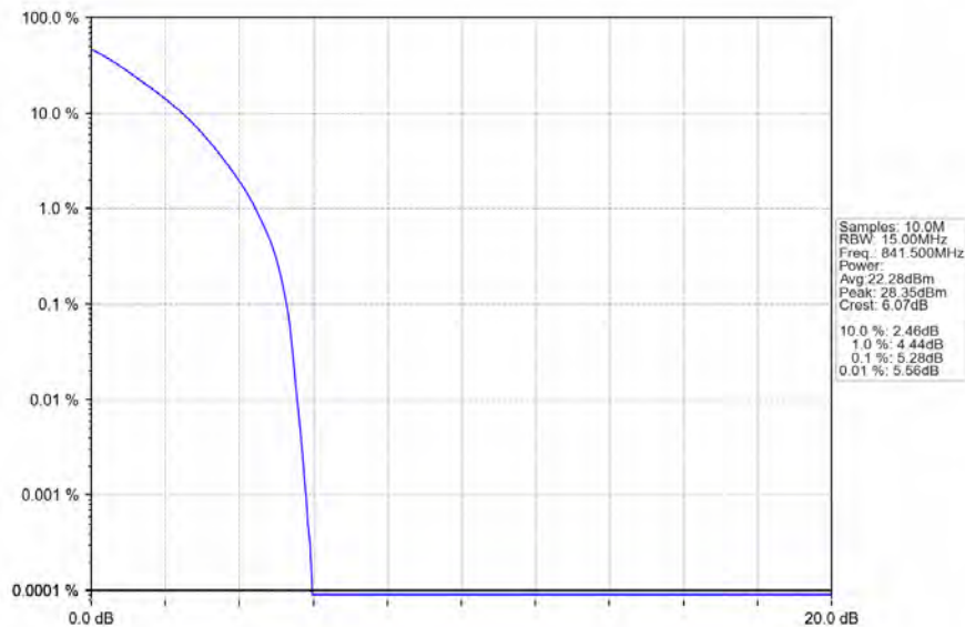
Band26c_15MHz_QPSK_HCH_841.5MHz_RB_75_0_NTNV
