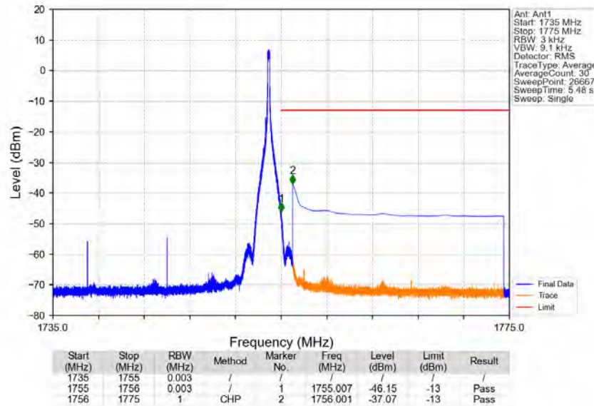
Band4_20MHz_QPSK_HCH_1745MHz_RB_1_99_NTNV
