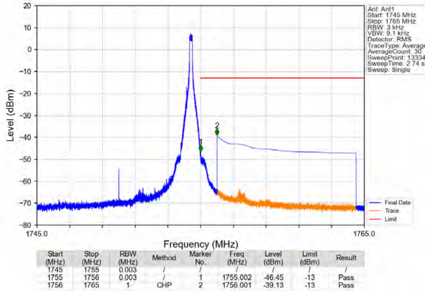
Band4_10MHz_QPSK_HCH_1750MHz_RB_1_49_NTNV
