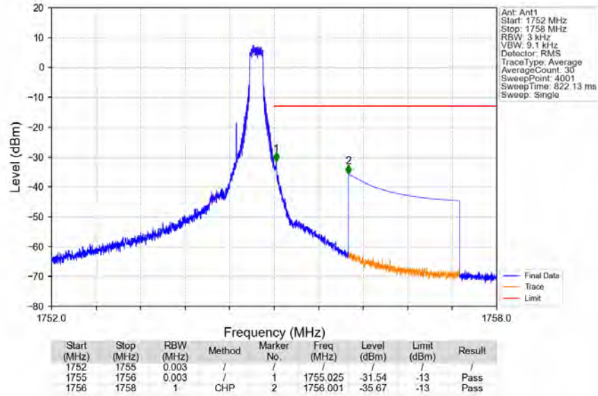
Band4_3MHz_QPSK_HCH_1753.5MHz_RB_1_14_NTNV
