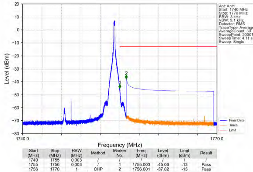
Band4_15MHz_QPSK_HCH_1747.5MHz_RB_1_74_NTNV
