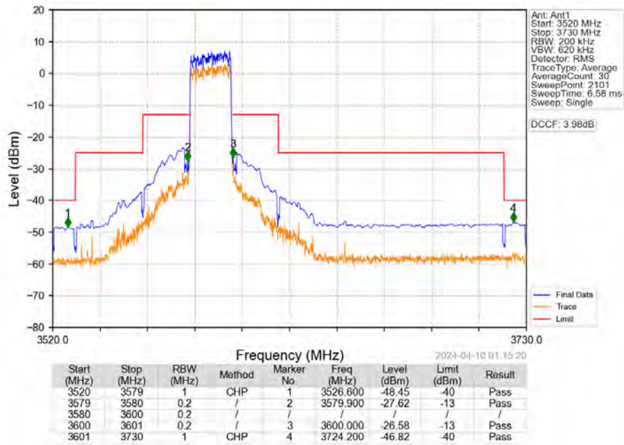
Band42c_20MHz_16QAM_LCH_3560MHz_RB_1_0_NTNV
