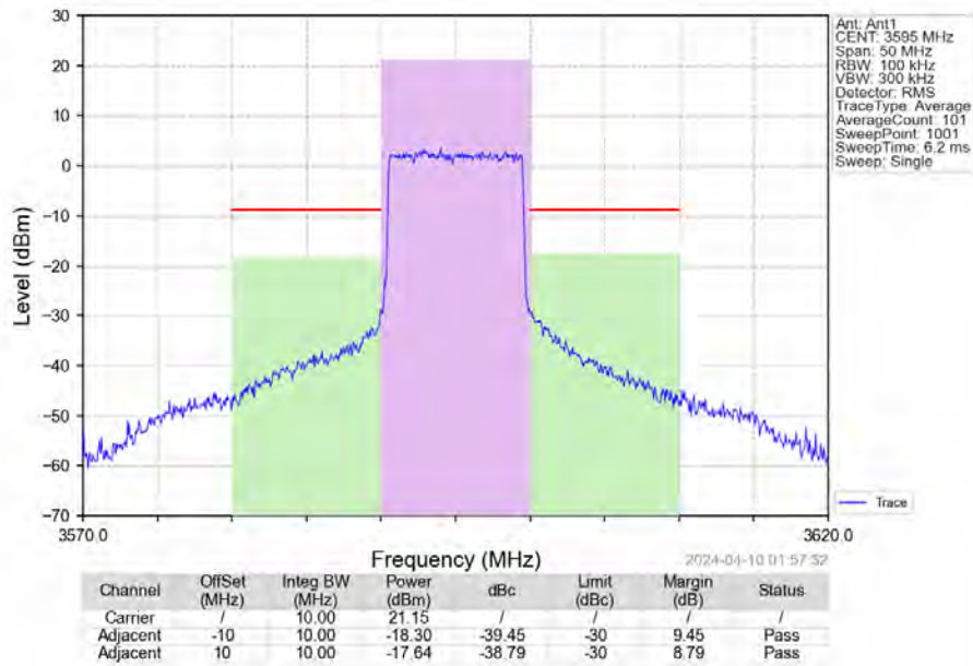
Band42c_10MHz_QPSK_HCH_3595MHz_RB_50_0_NTNV
