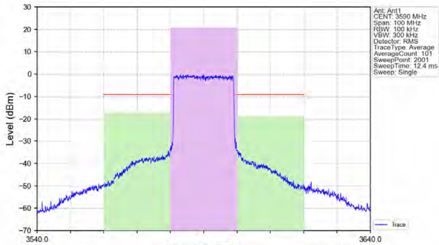
Band42c_20MHz_QPSK_HCH_3590MHz_RB_100_0_NTNV
