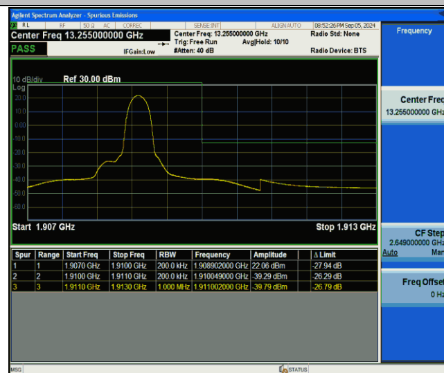
Band2-20MHz-QPSK-19100-1RB#99-PASS
