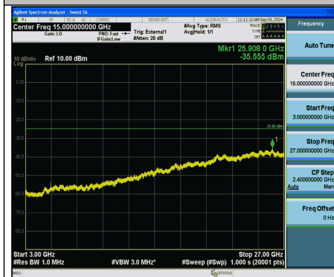
Band41-20MHz-QPSK-41490-1RB#0-3000~27000-PASS
