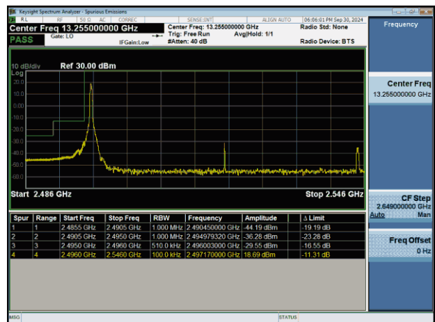
NTNV-n41-PC2-30-50-L-DFT-BPSK-Edge_1RB_Left-PASS
