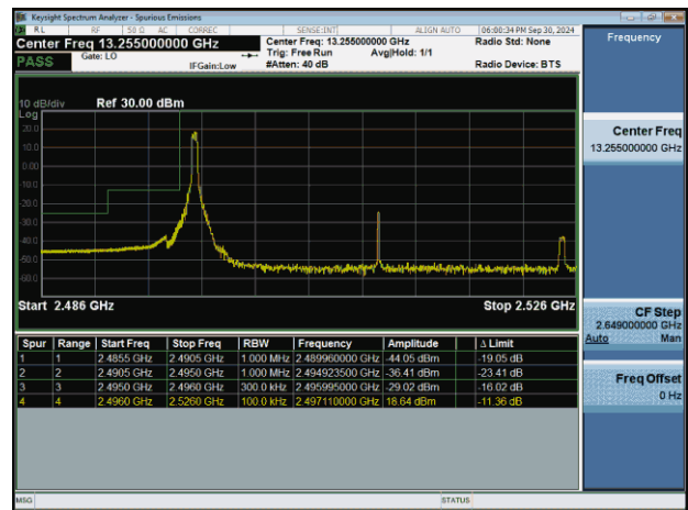
NTNV-n41-PC2-30-30-L-CP-QPSK-Edge_1RB_Left-PASS
