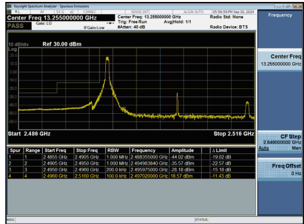
NTNV-n41-PC2-30-20-L-CP-QPSK-Edge_1RB_Left-PASS
