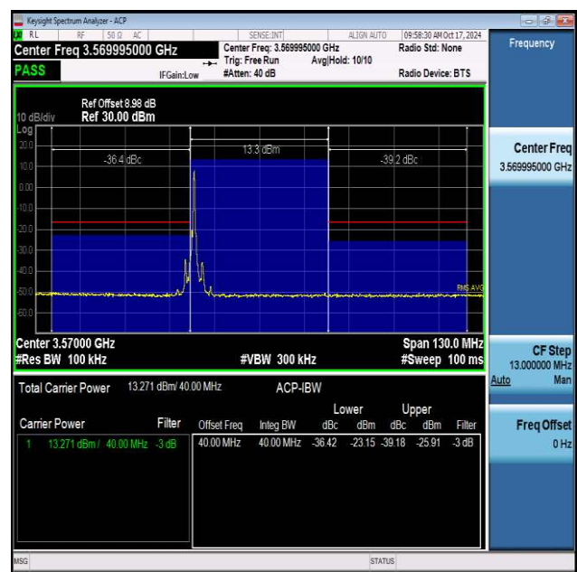
NTNV_N48_PC3_30_40_L_TID2_#1_+40_40
