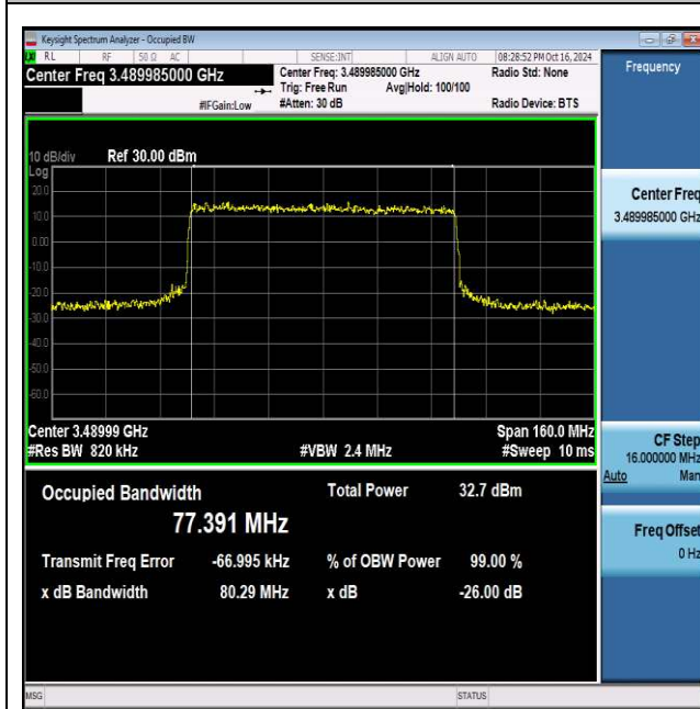
NTNV_N77-3450-3550_PC2_30_80_L_TID7_Ant1#1
