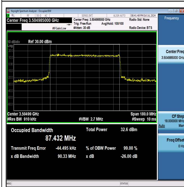
NTNV_N77-3450-3550_PC2_30_90_H_TID7_Ant1#1
