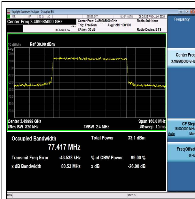
NTNV_N77-3450-3550_PC2_30_80_L_TID5_Ant1#1
