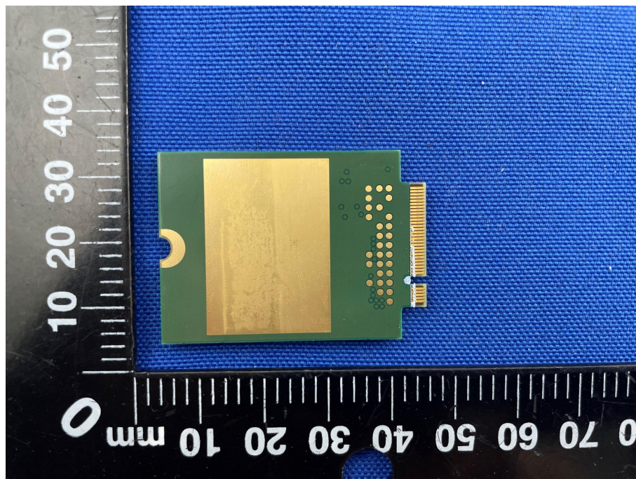
RF MODULE REAR VIEW -FM101-GL
