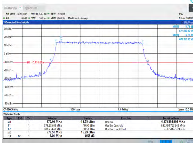
Band71-5MHz-QPSK-133297-25RB#0
