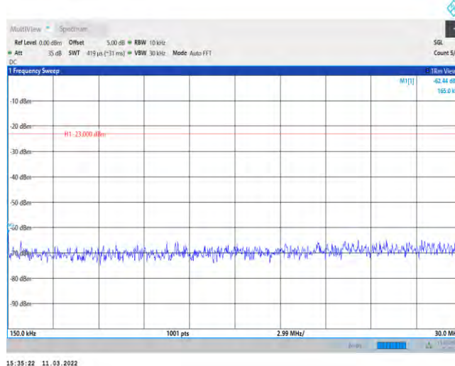
Band71-20MHz-QPSK-133222-1RB#0-Range2:0.15~30MHz
