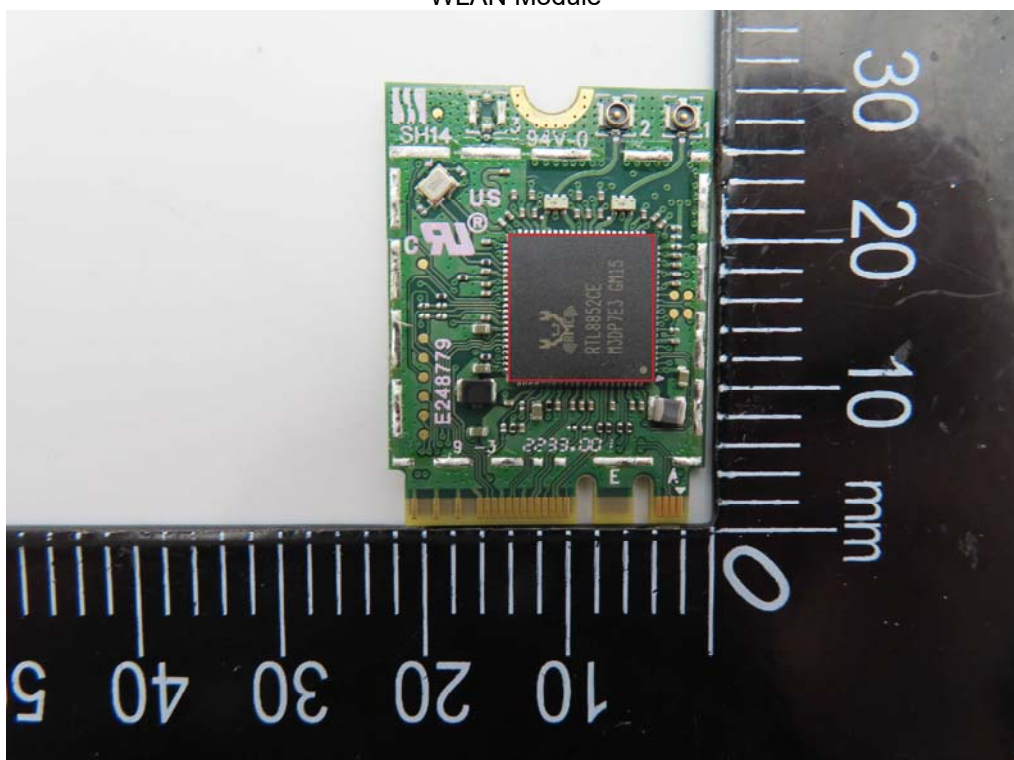
WLAN Module
