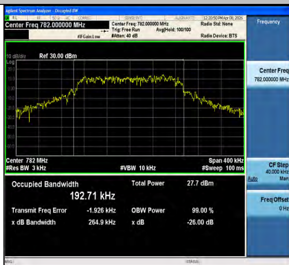
Band13-0.18-BPSK-23230-PASS
