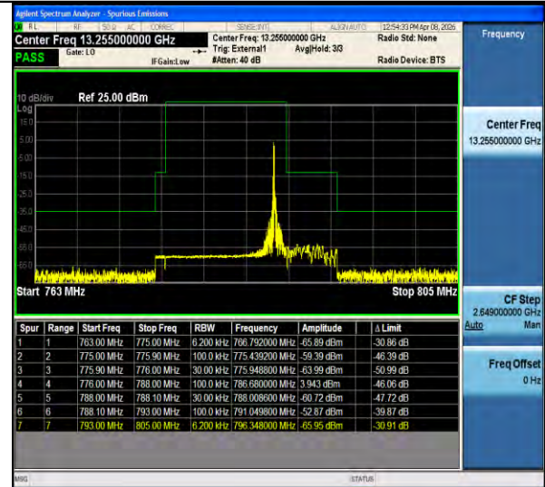
Band13-0.18-BPSK-23278-PASS
