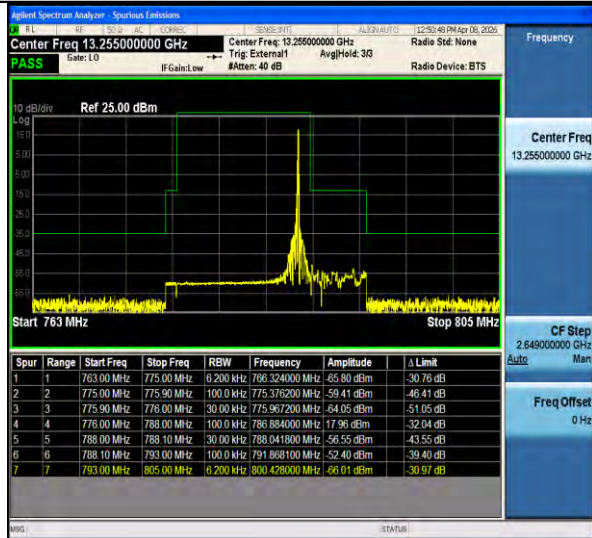
Band13-0.18-BPSK-23278-PASS
