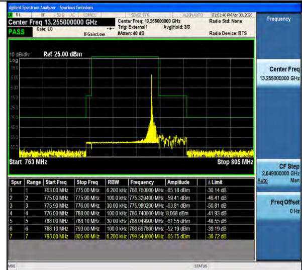
Band13-0.18-BPSK-23278-PASS
