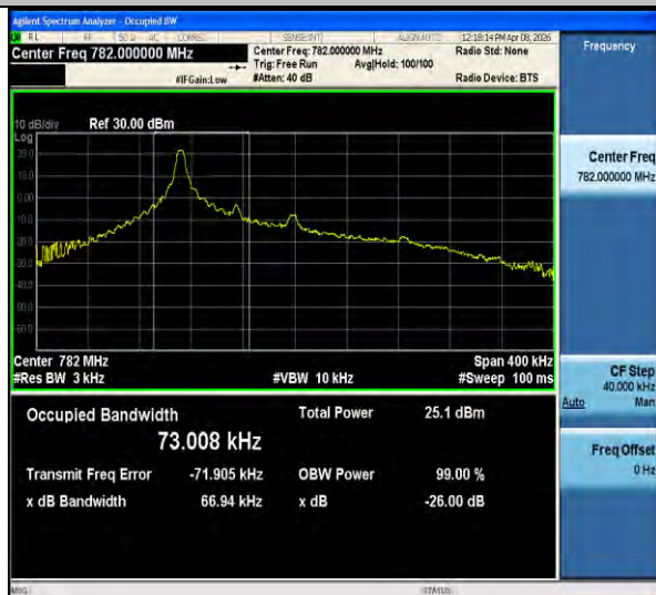
Band13-0.18-BPSK-23230-PASS
