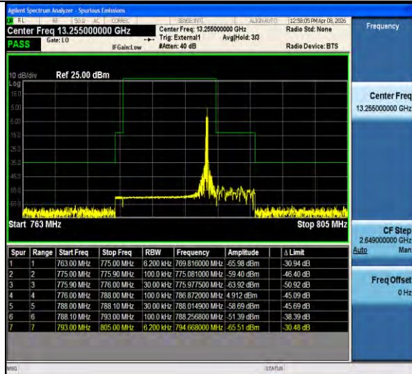
Band13-0.18-BPSK-23278-PASS
