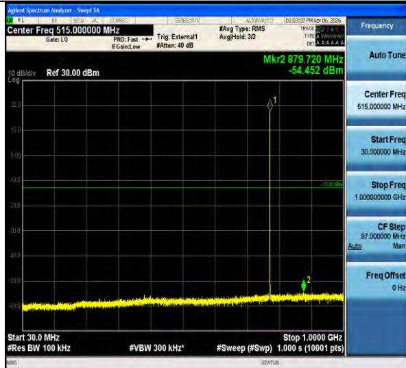
Band13-0.18-BPSK-23182-763-775-PASS
