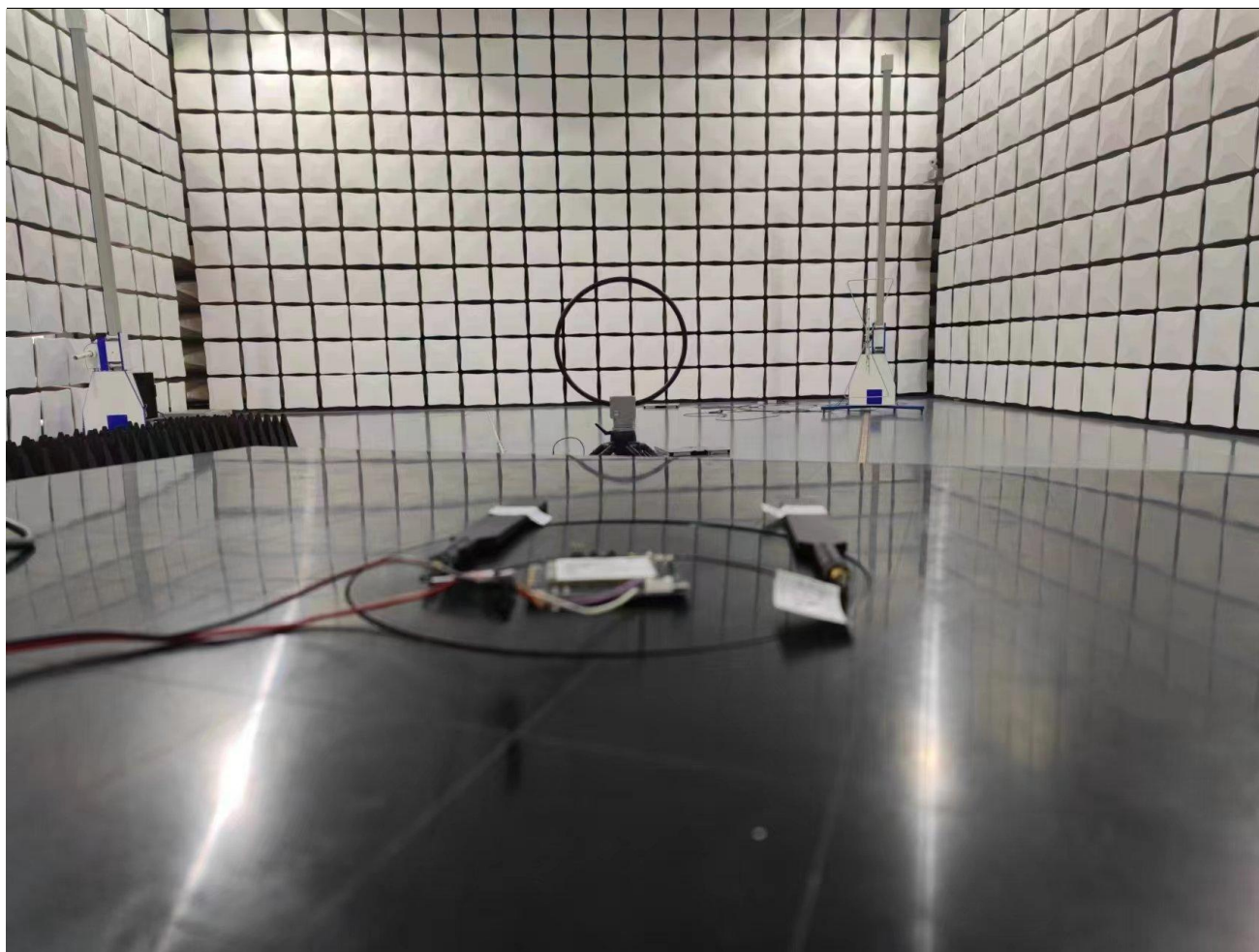
9KHz~30MHz
