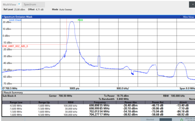
Band12-3MHz-QPSK-23165-1RB#14
