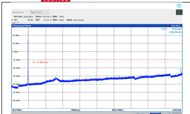
Band71-10MHz-QPSK-133297-1RB#0-Range:30~6990MHz
