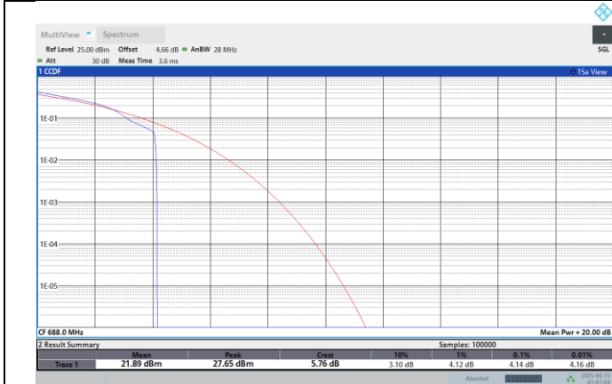
Band71-20MHz-16QAM-133372-1RB#0
