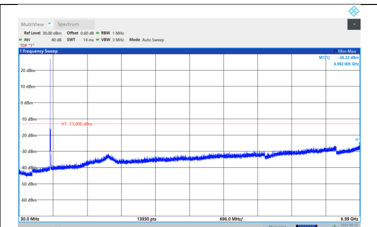
Band71-10MHz-QPSK-133422-1RB#0-Range:30~6990MHz
