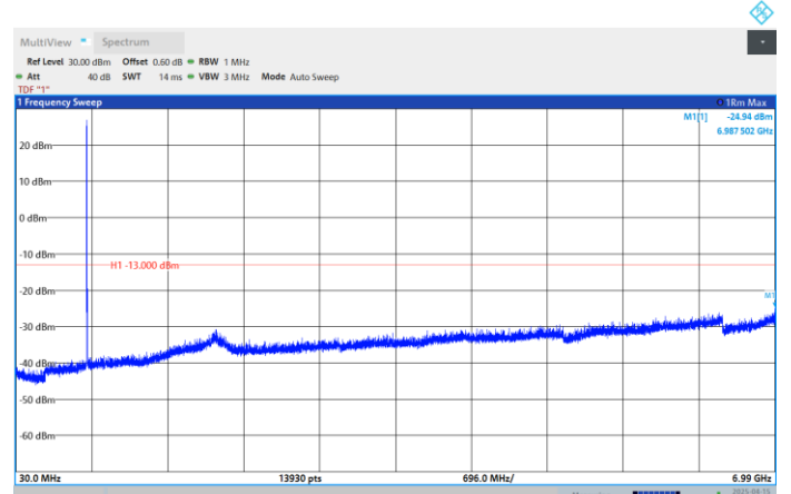
Band71-10MHz-QPSK-133172-1RB#0-Range:30~6990MHz
