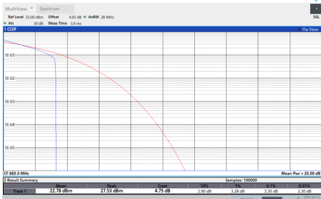
Band71-20MHz-QPSK-133372-1RB#0
