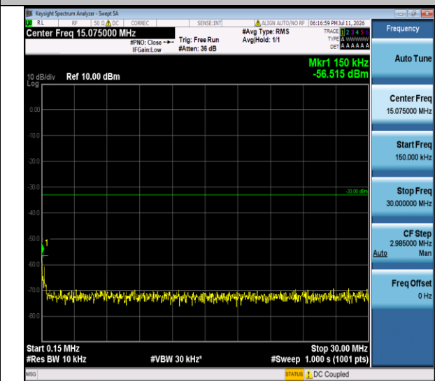
Band II-9538-0.15~30MHz-PASS
