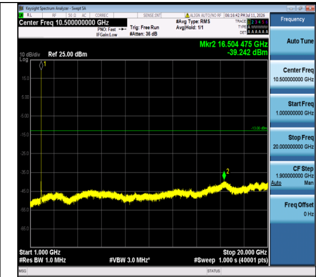
Band II-9400-1000~20000MHz-PASS
