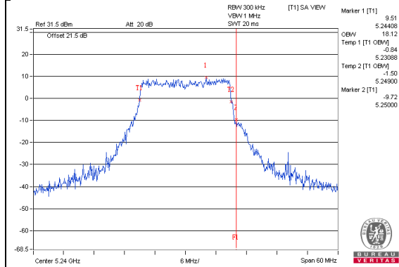
802.11ac(VHT20)_Chain2 / CH48
