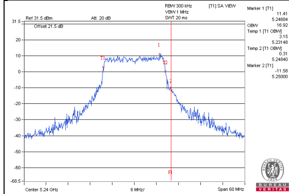
802.11a_Chain2 / CH48
