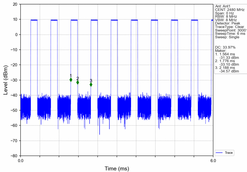
2M_HCH_2480MHz_Ant1_NTNV
