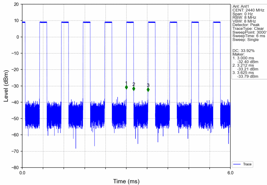
2M_MCH_2440MHz_Ant1_NTNV
