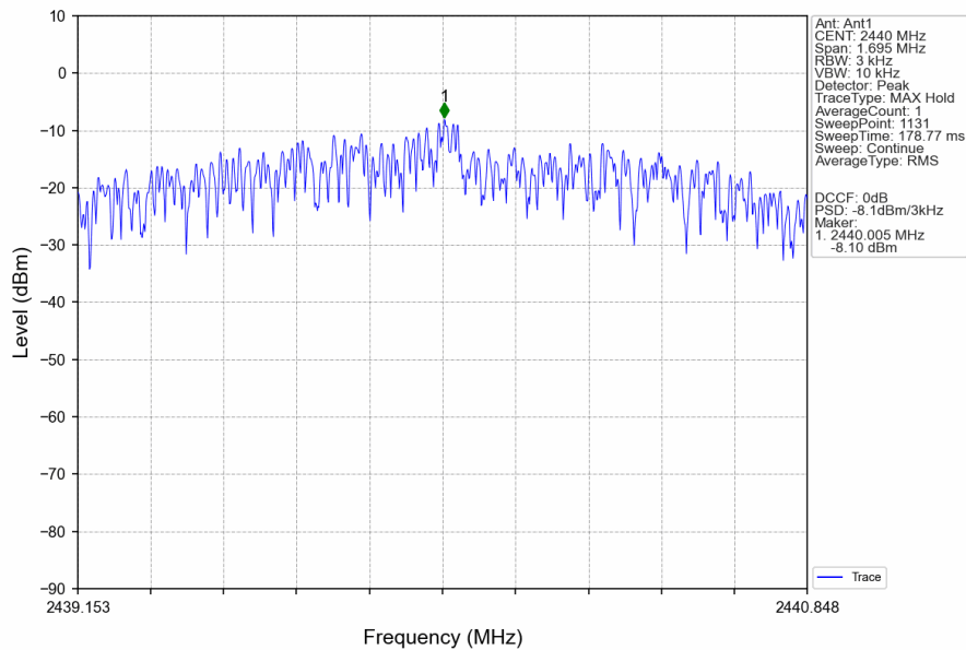
2M_MCH_2440MHz_Ant1_NTNV
