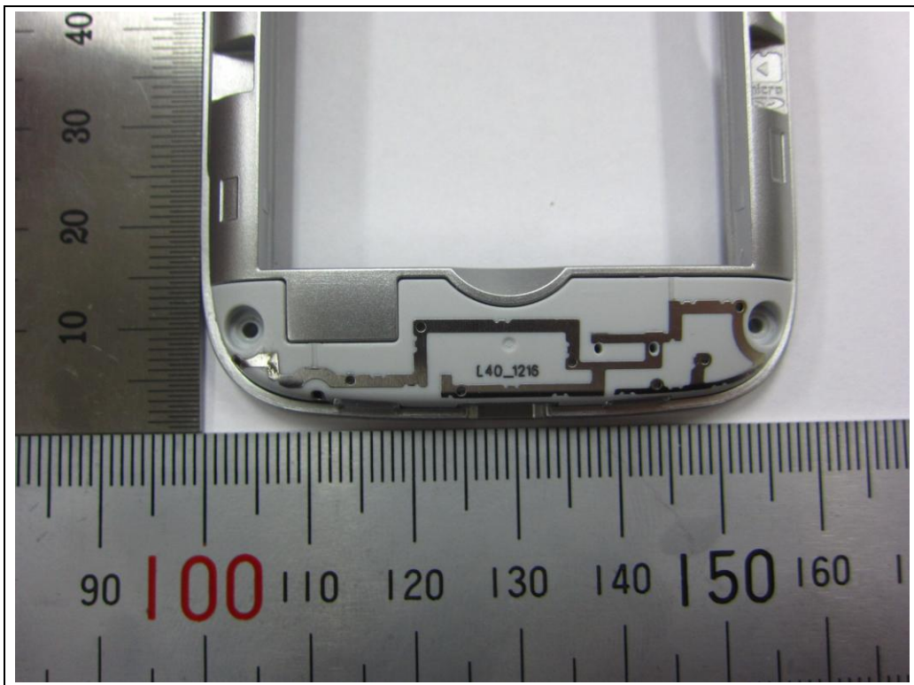
<GSM Antenna>
