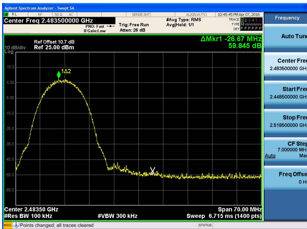
Band Edge (802.11b-CH11)
