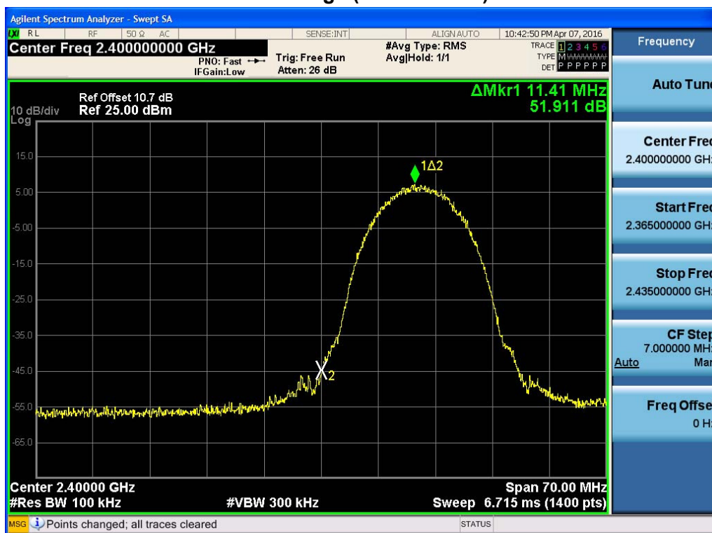
Band Edge (802.11b-CH1)
