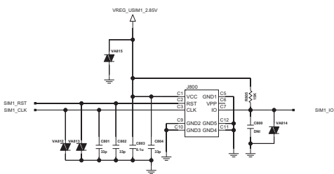
USIM Socket
