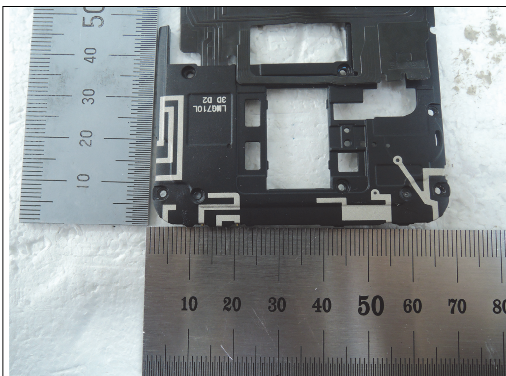
<Antenna 3>
