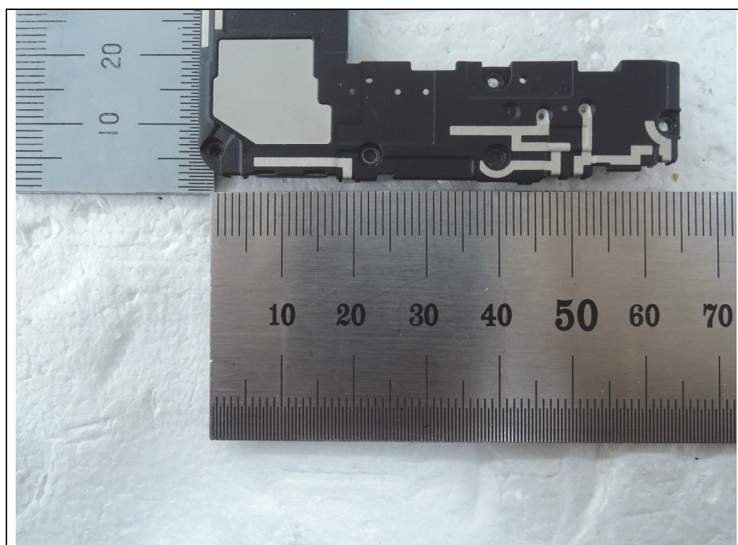
<Antenna 1>
