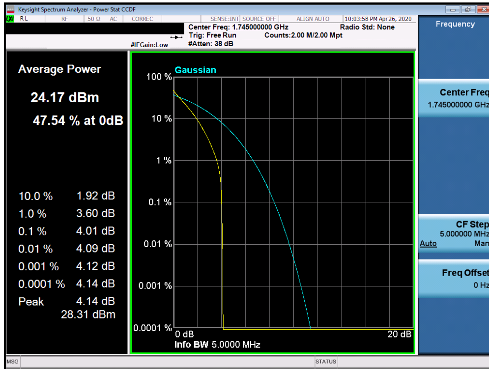
Plot 7-581. PAR Plot (5G sub6 n66/4 - 5.0MHz BPSK - Full RB Configuration)
