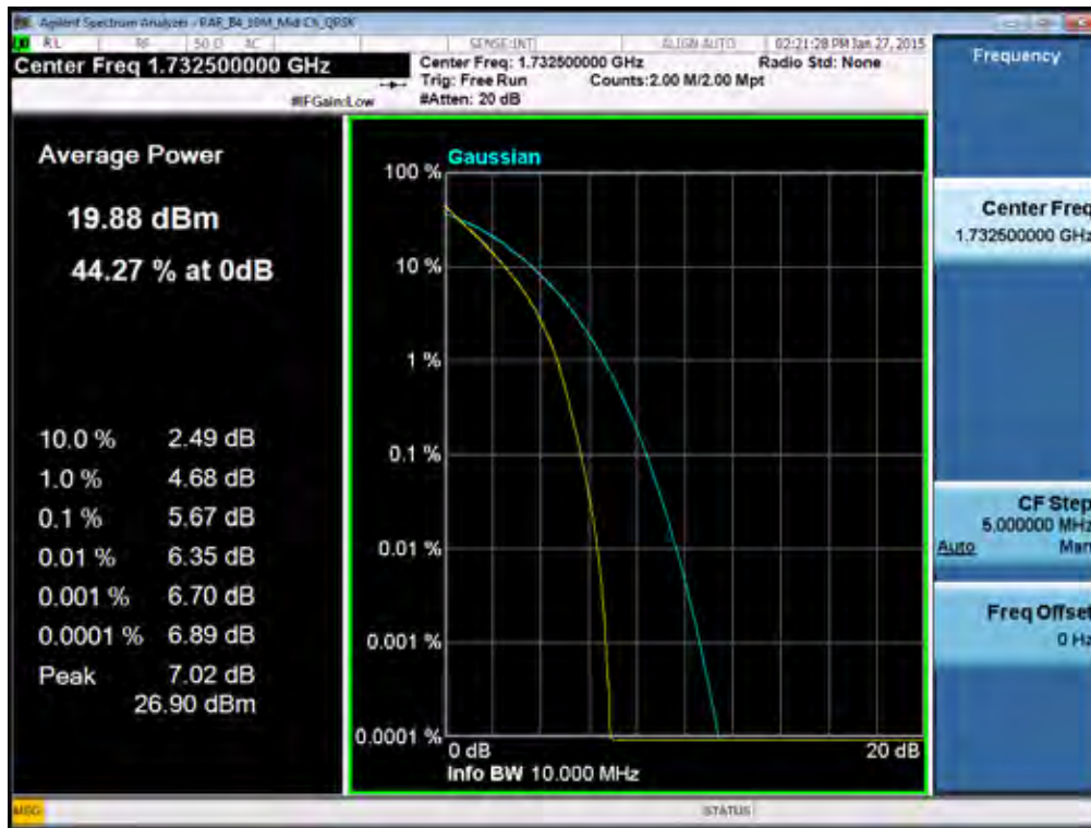
BAND 4. PAR Plot (10M BW_Ch.20175_QPSK_RB50_0)
