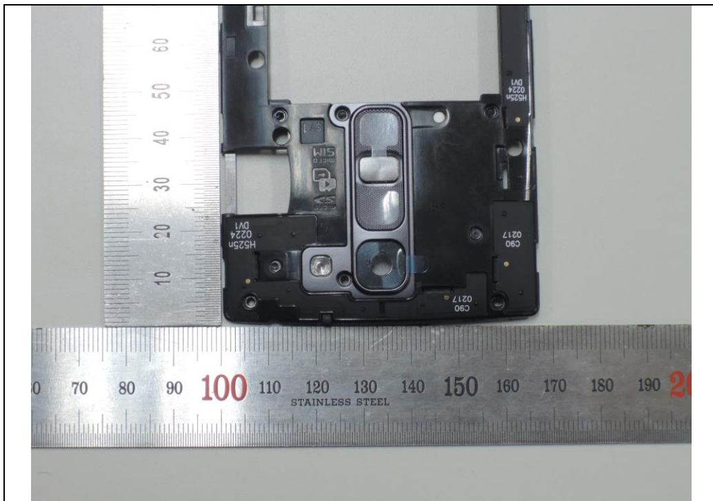
WLAN_BT_GNSS_LTE ANT
