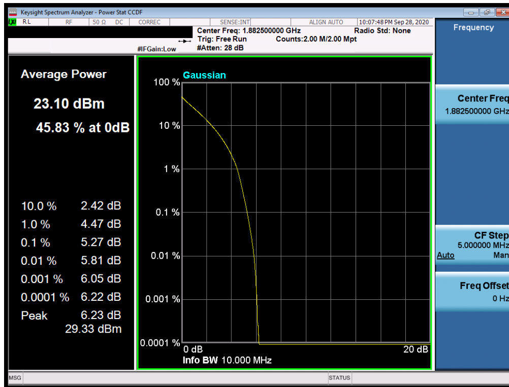
Plot 7-105. PAR Plot (LTE Band 25/2 - 10MHz QPSK - Full RB Configuration)
