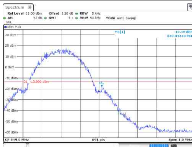
GSM850_251
