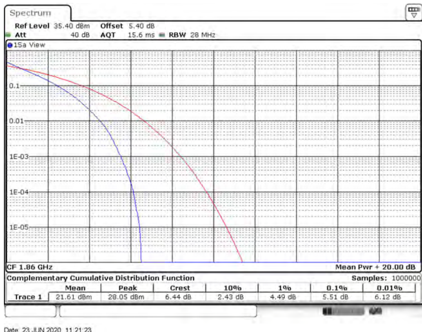
Band2-20MHz-QPSK-18700-100RB#0
