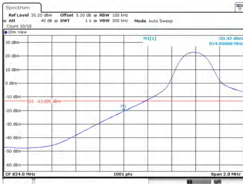
Band5-10MHz-QPSK-20450-1RB#0
